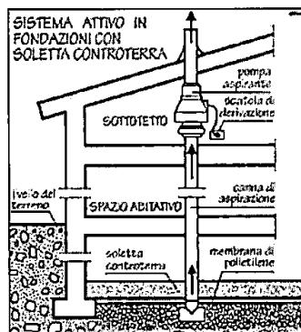
Fig.3 Sistema attivo.
